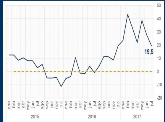
Gráfico 1: EE.UU. - Índice de condiciones del sector manufacturero (En puntos)
