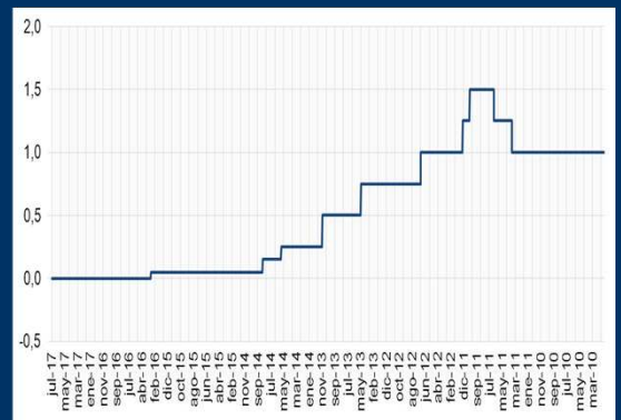
Gráfico 2: Zona Euro - Tasa de política monetaria (En porcentaje)
