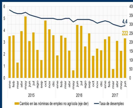
Gráfico 1: EE.UU. - Indicadores del mercado laboral (En porcentaje y miles)
