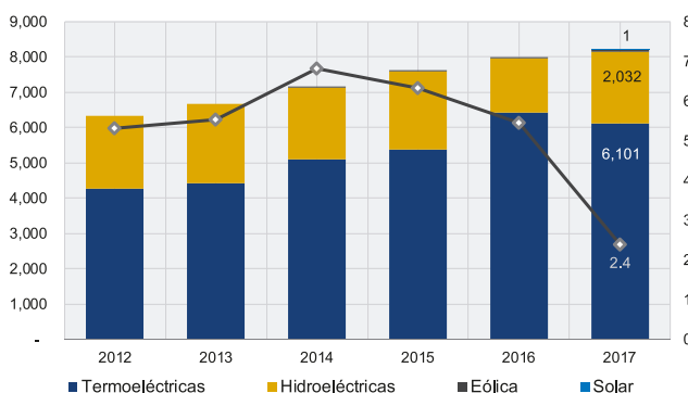
Gráfico 3.17: Generación de energía eléctrica por fuente** (En GWh y crecimiento interanual en porcentaje)
