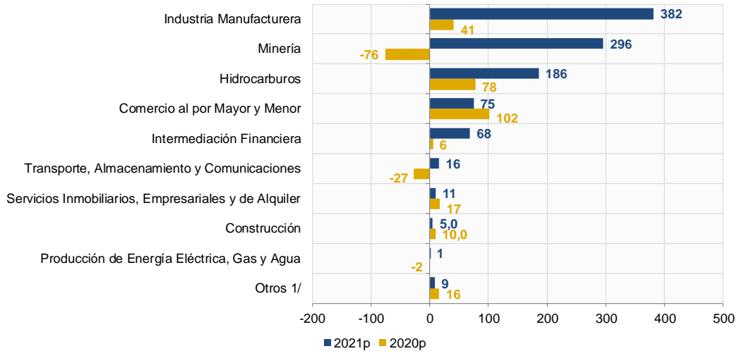
Gráfico 1: IED bruta por actividad económica, 2020 - 2021 (En millones de dólares estadounidenses)
