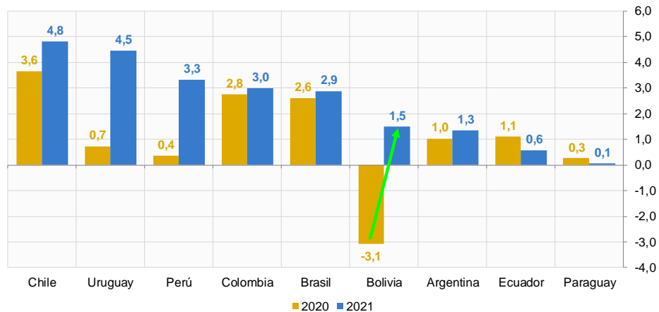
Gráfico 2: Flujos de IED Neta de países de América del Sur, 2020 - 2021 (En porcentaje del PIB)
